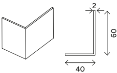
Winkelprofil 40/60/2
