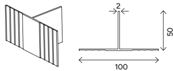
T-Profil 100/50/2
