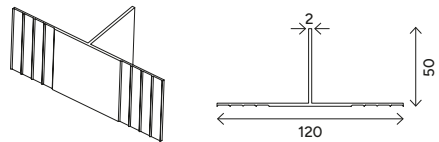
T-Profil 120/50/2
