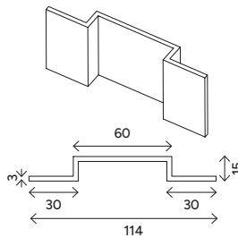
Hutprofil 30/15/60/15/30-3mm in Längen á 6000 mm
