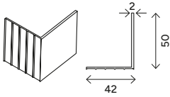
Winkelprofil 42/50
