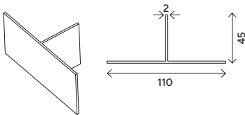
T-Profil 110/45/2
